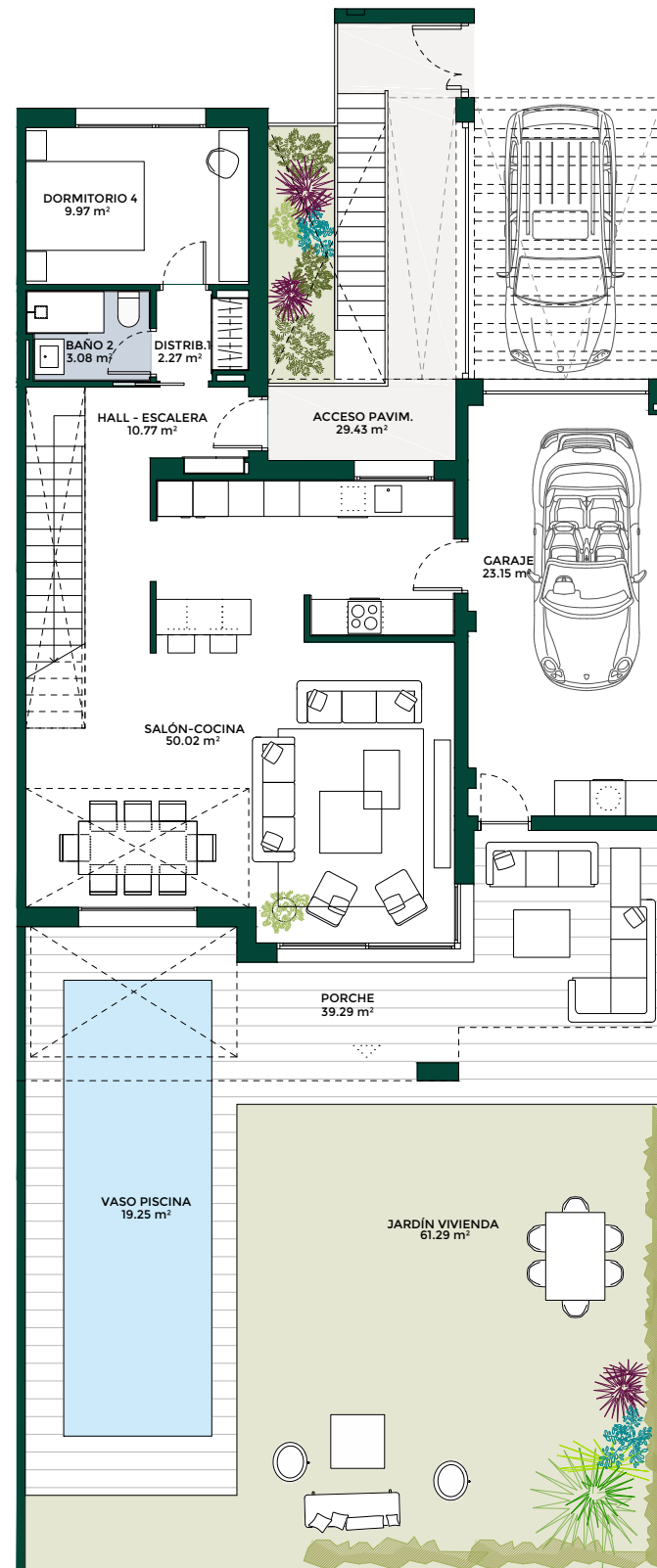
PLANTA BAJA
